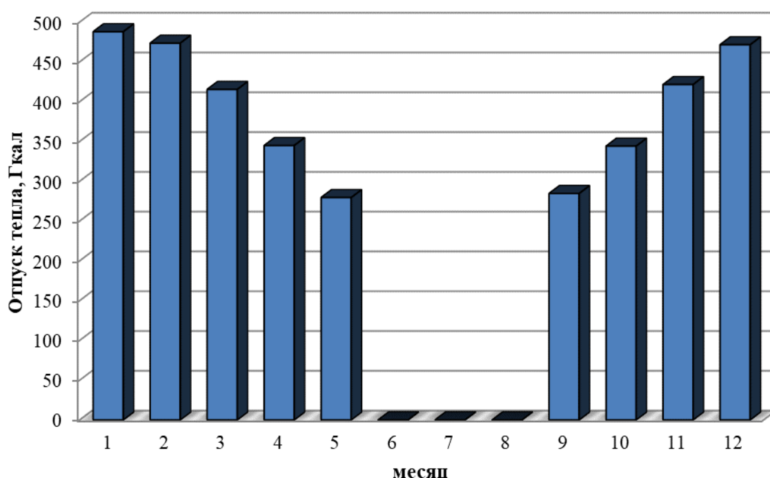
Рисунок 1.2 – Оптимальный температурный график отпуска тепловой энергии для котельной «Поселковая» Новокусовского сельского поселения
