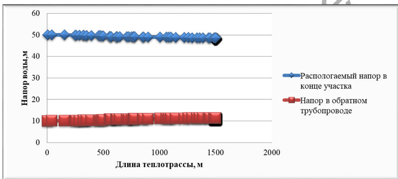
Рисунок 2.7 – Пьезометрический график тепловой сети котельной «Поселковая» с. Ново-Кузово по магистральному выводу
