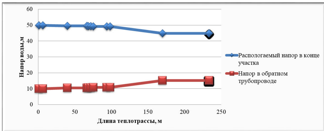
Рисунок 2.8 – Пьезометрический график тепловой сети котельной «Школьная» с. Ново-Кусково по магистральному выводу
