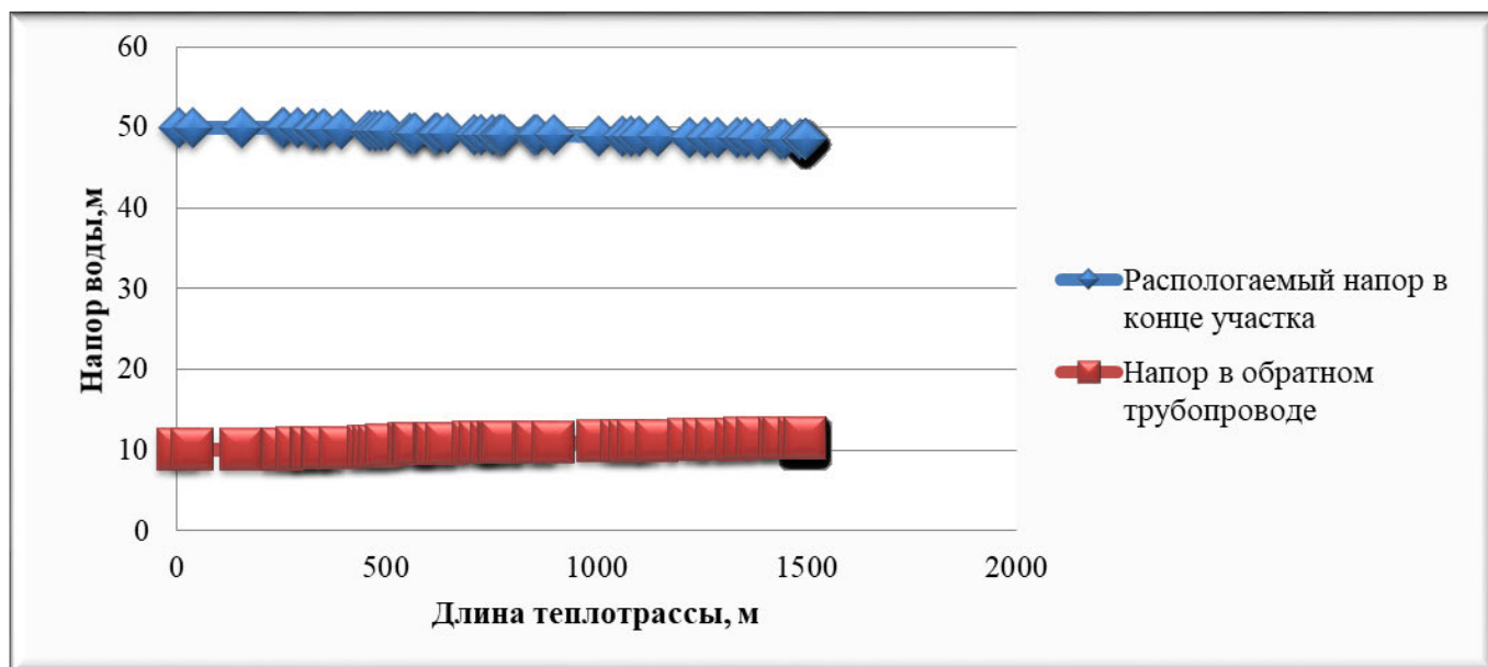
Рисунок 2.5 – Пьезометрический график тепловой сети котельной «Поселковая» с. Ново-Кузово по магистральному выводу
