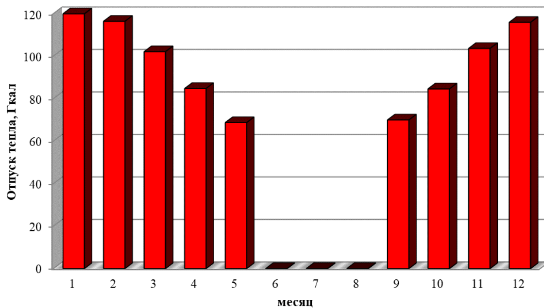
Рисунок 1.3 – Оптимальный температурный график отпуса тепловой энергии для котельной «Школьная» Новокусовского сельского поселения
