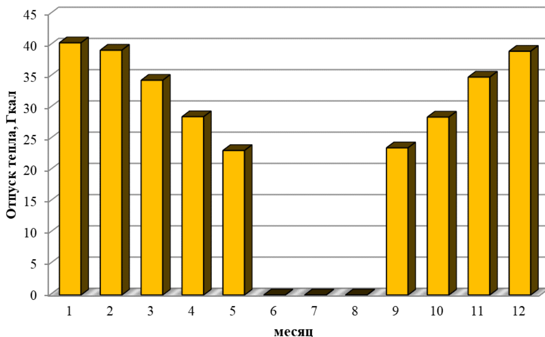
Рисунок 1.5 – Оптимальный температурный график отпуса тепловой энергии для котельной с. Казанка Новокусовского сельского поселения
