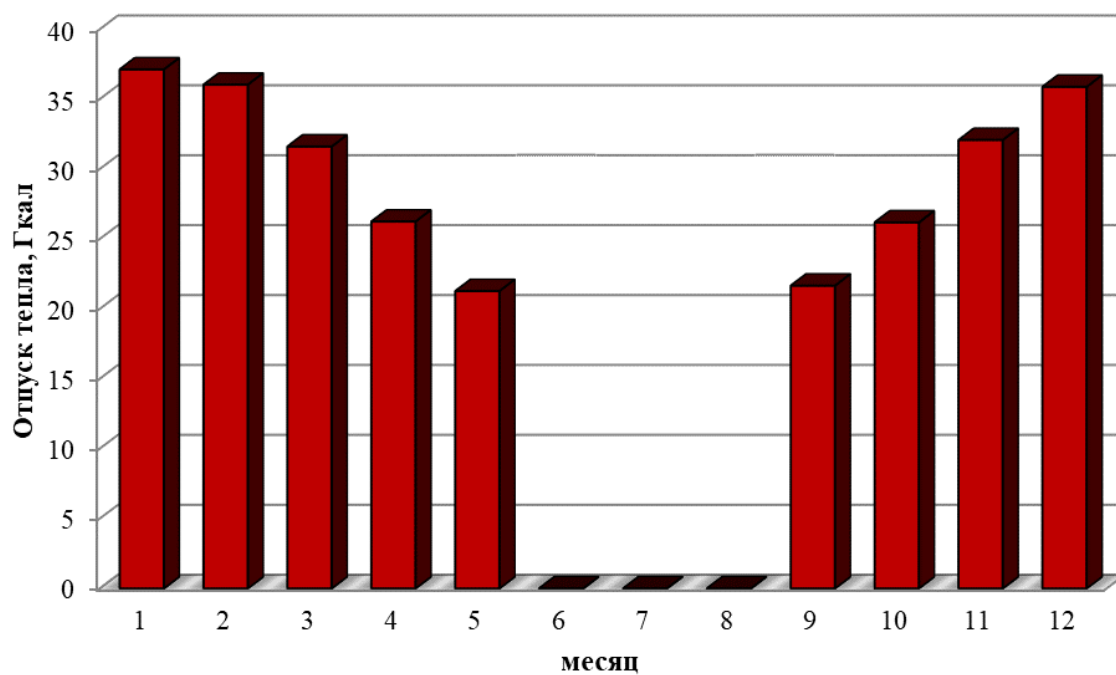
Рисунок 1.4 – Оптимальный температурный график отпуса тепловой энергии для котельной с. Казанка Новокусовского сельского поселения
