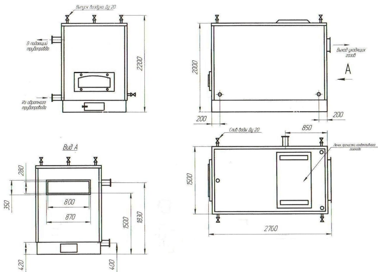
Рисунок 2.1 – Котел КВР 0,5 КБ
