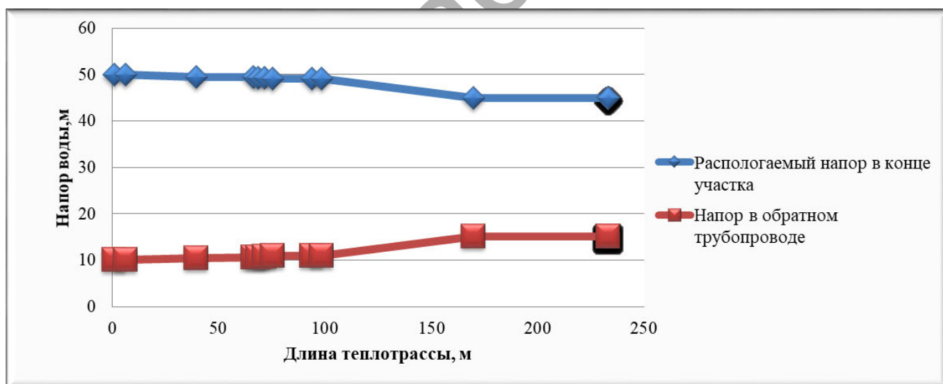
Рисунок 2.6 – Пьезометрический график тепловой сети котельной «Школьная» с. Ново-Кузово по магистральному выводу
