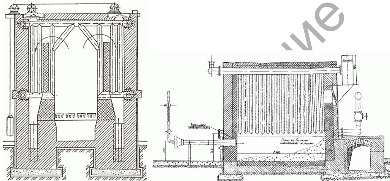
Рисунок 2.2 – Поперечный и продольный разрез котла НР-18
